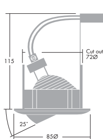
Tiltable +/- 25°
